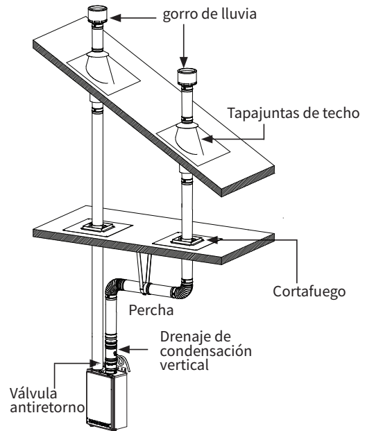
Instalación Vertical
