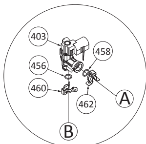
Sección Bypass TKGU-38-IN/EN
