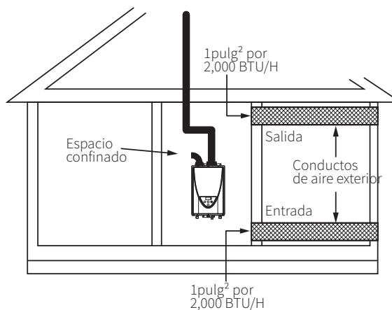
Fig. 4- Aberturas de conductos horizontales
