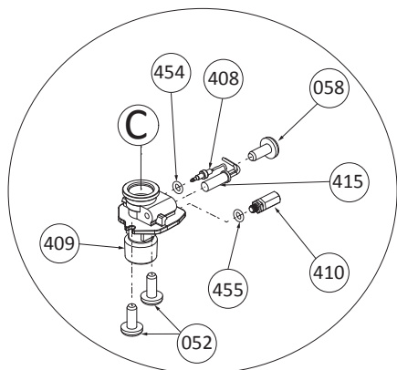
Sección de salida de agua
