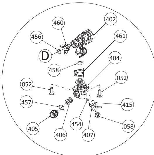
Sección de entrada de agua
