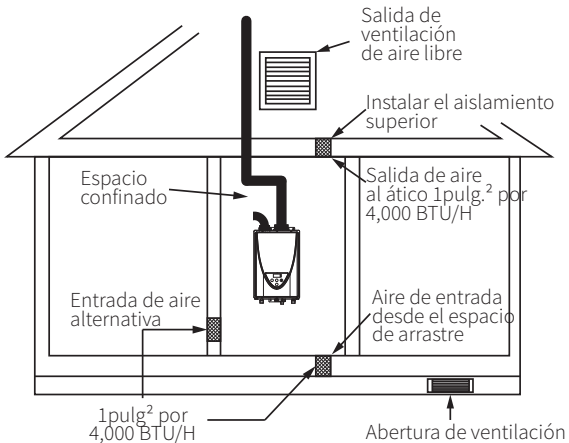
Fig. 1- Directo a las aberturas de aire libre
