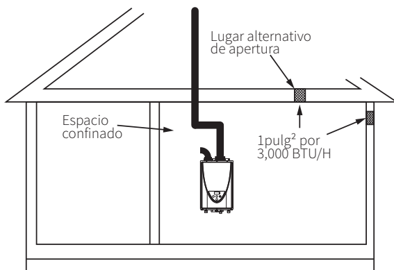
Fig. 5- Abertura sola
