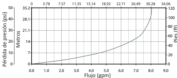
Pérdida de presión Flujo (lpm)
