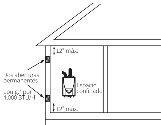
Fig. 2- Directo a las aberturas de aire libre Dos aberturas permanentes
