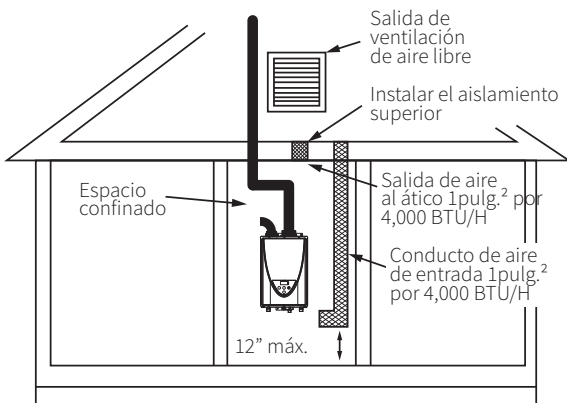
Fig. 3- Aberturas de conductos verticales
