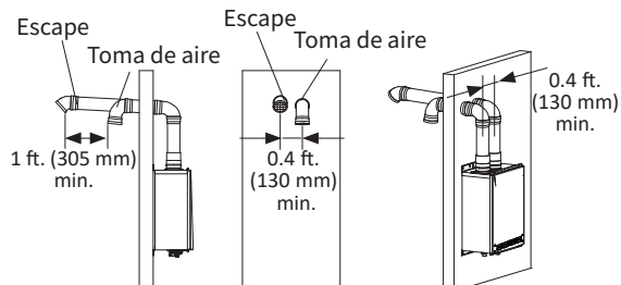
Instalación de pared lateral de ventilación directa
