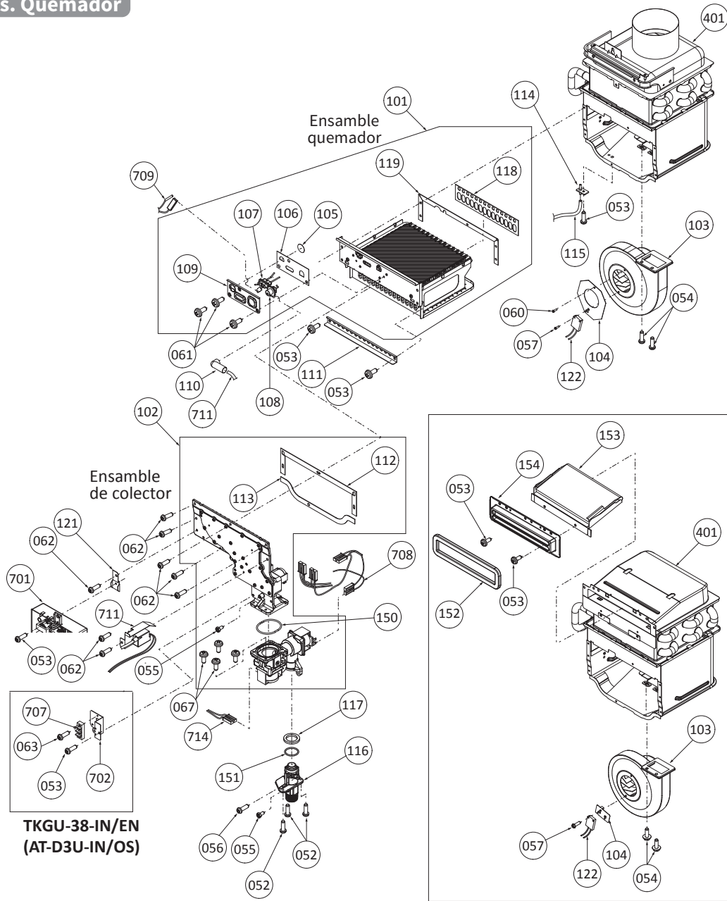
Sección de escape (modelo exterior)
