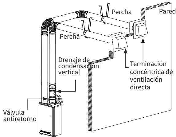
Instalación horizontal
