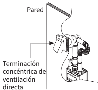
Instalación horizontal con terminación concéntrica de ventilación directa
