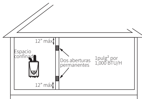
Fig. 6- Dos aberturas permanentes
