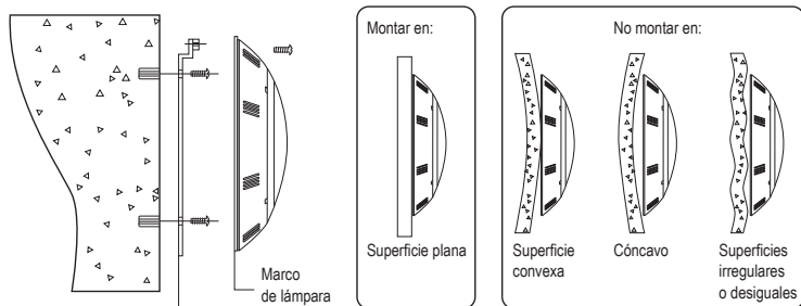
Figura 2. Montaje
